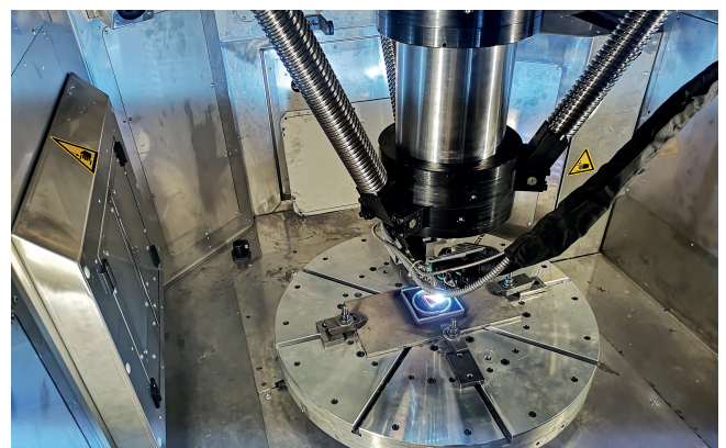
2 Lichtbogen-Auftragsschweißen mithilfe des eingewechselten Schweißmoduls © Metrom
